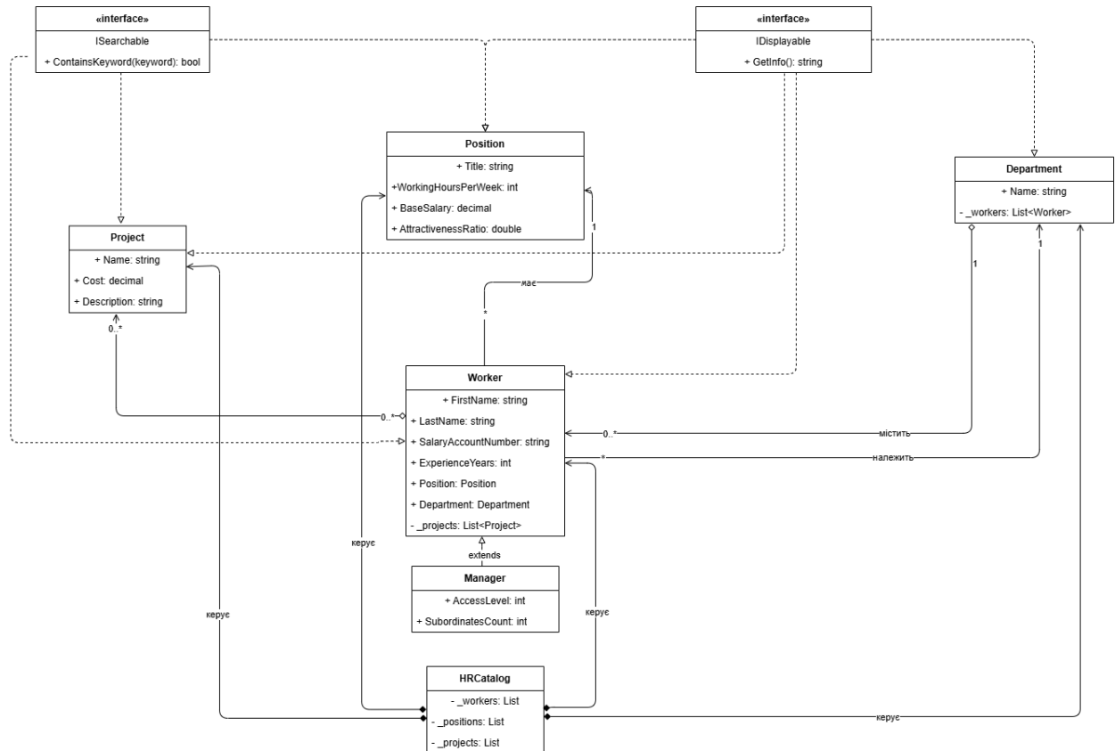
Рис.1 Діаграма класів
